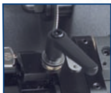
1 Sistema reversible de doble mordaza, a dos posiciones: a) duplicado de llaves de gorja. b) duplicado de llaves frontales.
